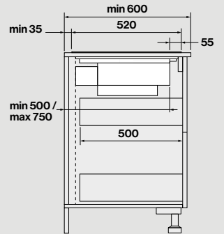
Vista laterale
