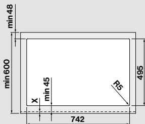
Dimensioni foro
