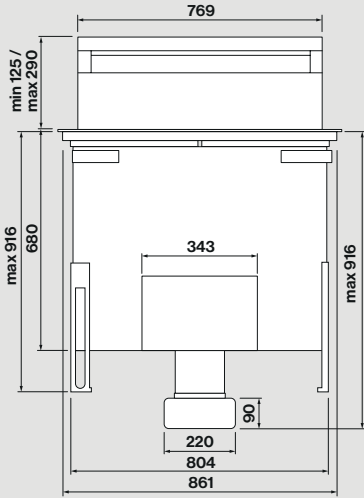
Vista frontale
