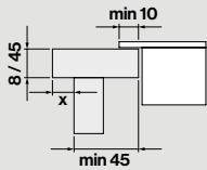
Dimensioni foro
