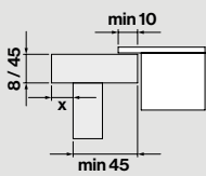
Dimensioni foro
