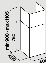
Parete telescopica
