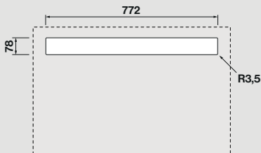
Dimensioni foro
