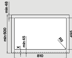
Dimensioni foro
