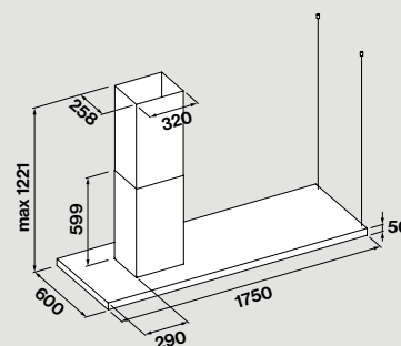
Versione sinistra
