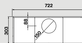
Vista superiore
