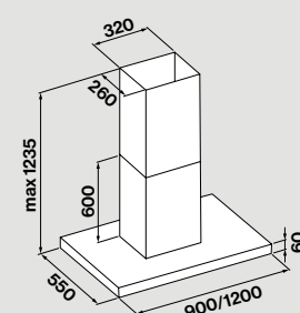
Isola
