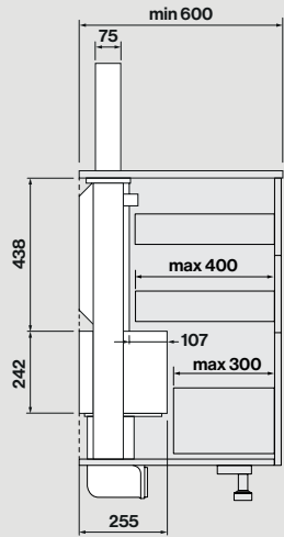
Dimensioni foro
