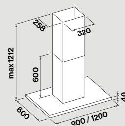
Isola
