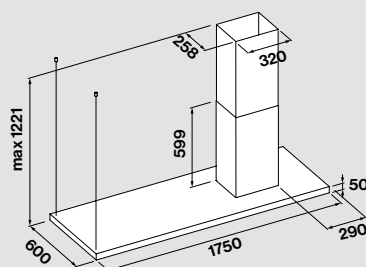
Versione destra
