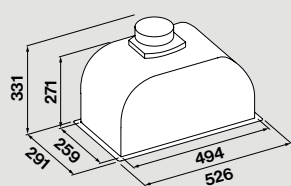
Foro per incasso 50 cm: 262 x 506 mm
