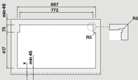
Dimensioni foro
