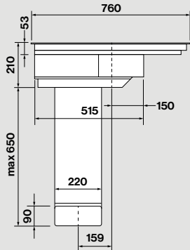
Vista frontale
