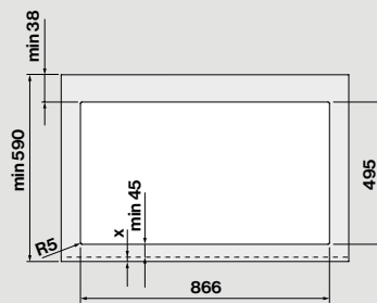
Dimensioni foro
