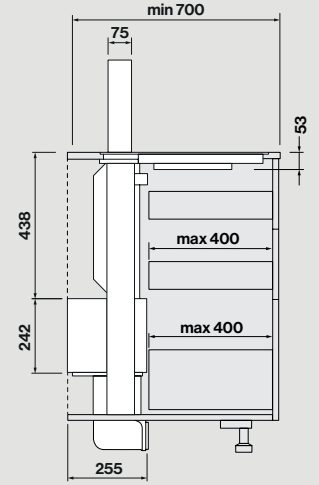
Vista laterale con motore in posizione posteriore
