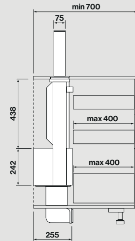
Vista laterale con motore in posizione posteriore
