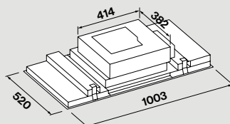
Foro per incasso 502 x 985 mm
