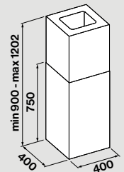
Isola
