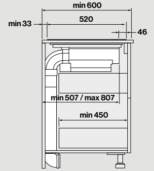
Vista laterale
