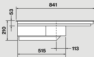
Vista frontale
