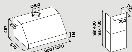
Camino opzionale
